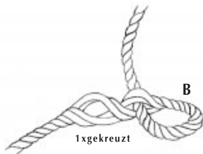
Abb. 5: Nun muss diese neu entstandene Schlaufe B fixiert werden. Dazu schaffen wir auf dem kürzeren Seilende (mit bereits bestehender Schlaufe A) eine weitere Öffnung, und zwar so, dass die 2 Litzenpaare nach der neuen Schlaufe B 1 mal gekreuzt bleiben.
